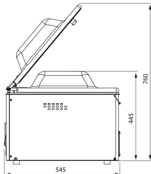
Wersja z wysoką pokrywą / Исполнение с высокой крышкой
